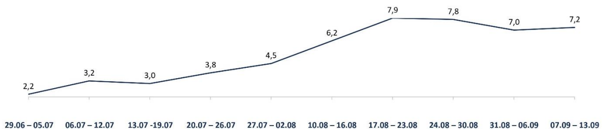
СРЕДНИЙ ИНДЕКС КОНФЛИКТОГЕННОСТИ, по неделям
